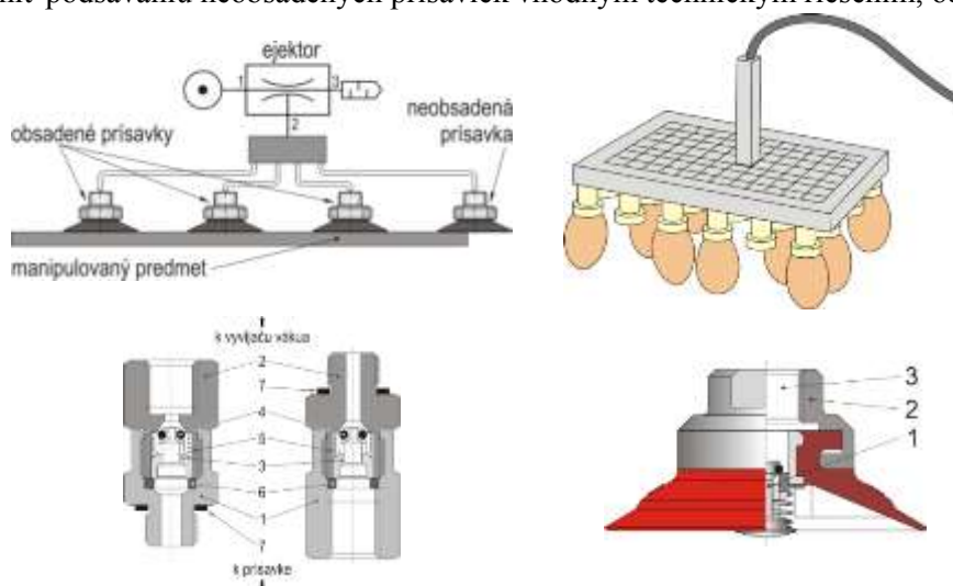
Obr. 7 Technické riešenia úspory vákuua – stlačeného vzduchu
