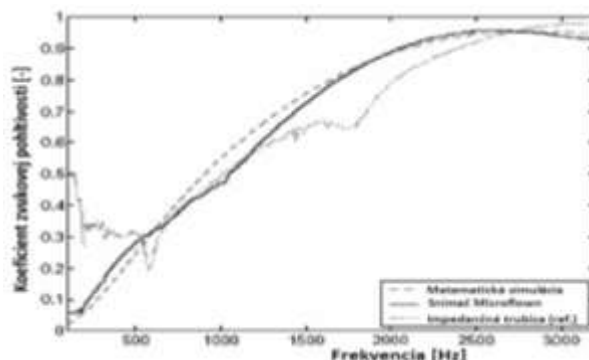
Obr. 3 Porovnanie výsledkov meraní koeficienta zvukovej pohltivosti [2]
