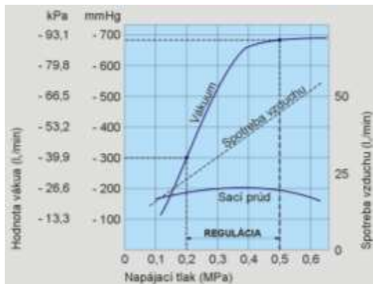
Obr. 3 Sacie funkcie ejektora
