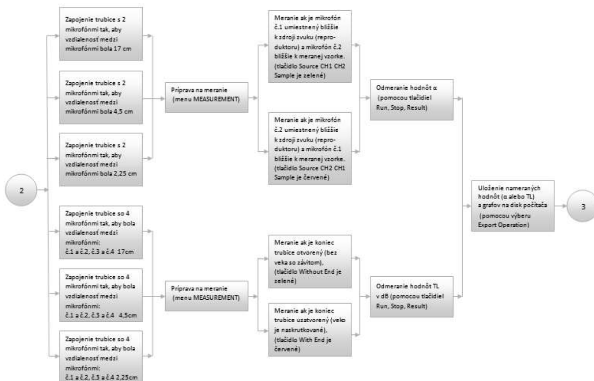
Obr. 4 Metodika merania vybraných akustických deskriptorov (pokračovanie)
