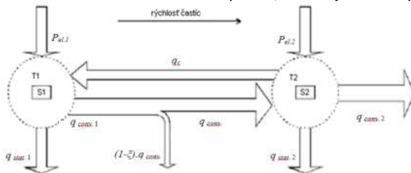
Obr. 1 Prehľad prúdenia tepla okolo snímača Microflown [6]
