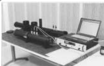
Obr. 1 Impedančná trubica
