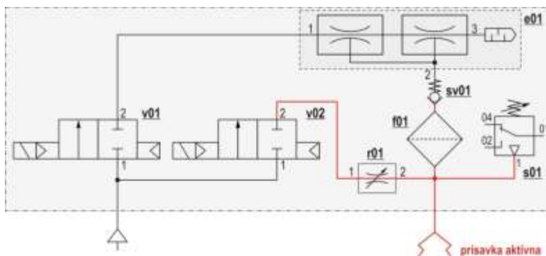
Obr. 6 Šetrenie stlačeného vzduchu správnym usporiadaním obvodu
