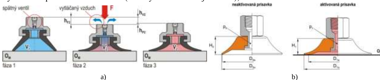
Obr. 2 Pasívna a aktívna prísavka
