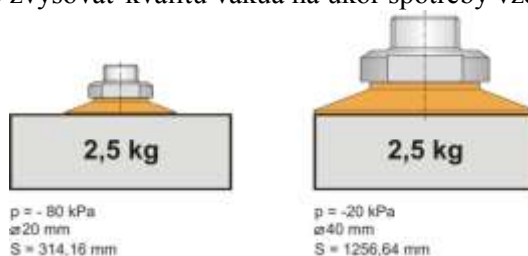
Obr. 4 Silové pomery na prísavke v závislosti na kvalite vákuu a veľkosti kontaktnej plochy prísavky s O_M
