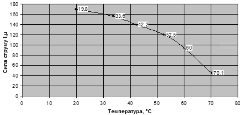
Рис. 1 Залежність сили струму від температури поверхні фотоелектричного модуля.
