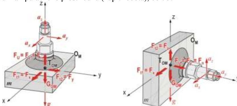
Obr. 5 Silové pomery na prísavke v závislosti od formy pôsobiacich zrýchlení
