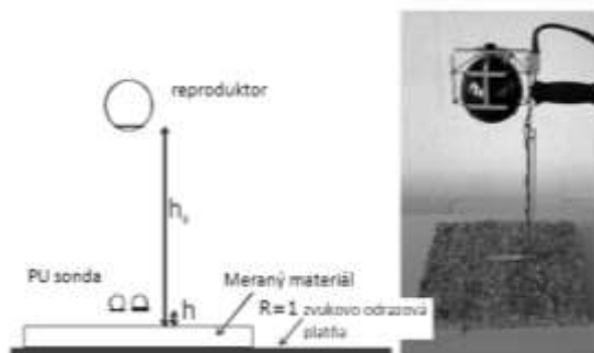
Obr. 2 Znáznornenie PU sondy a zariadenia [2]
